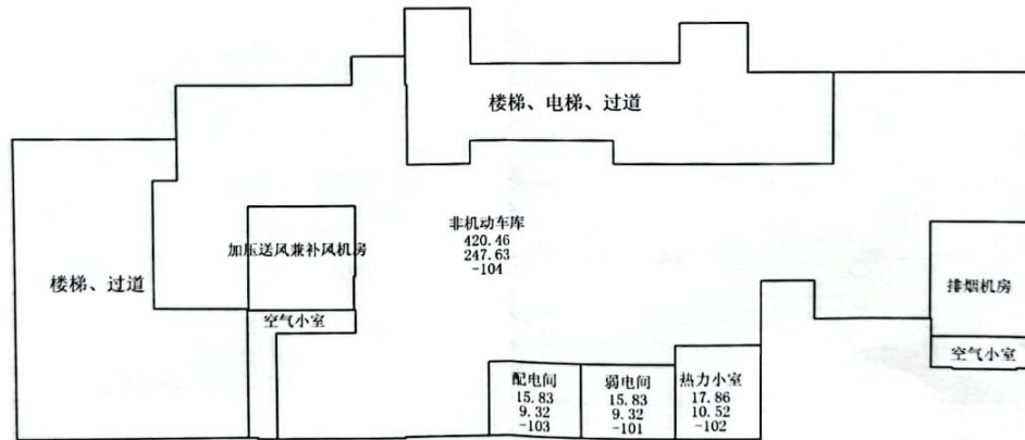
秦皇半岛六区29栋地下1层平面图
