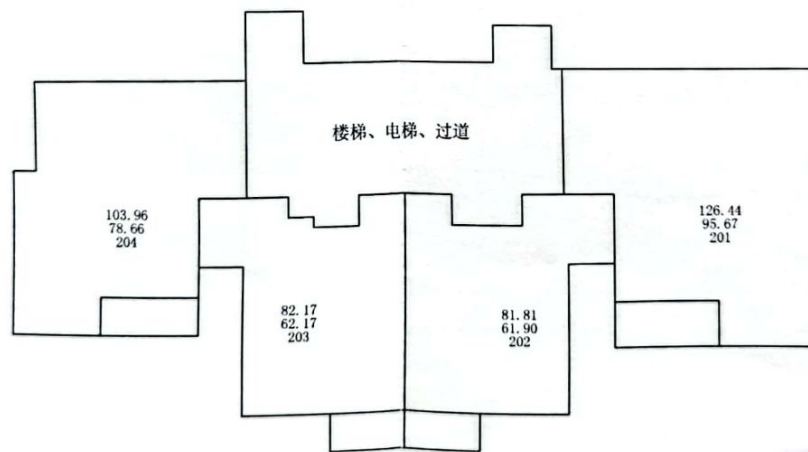
秦皇半岛六区29栋2-26层平面图
