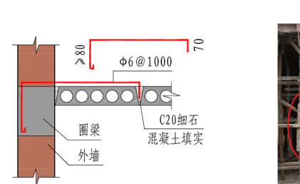
预制板侧面与外墙拉结 (✓)
