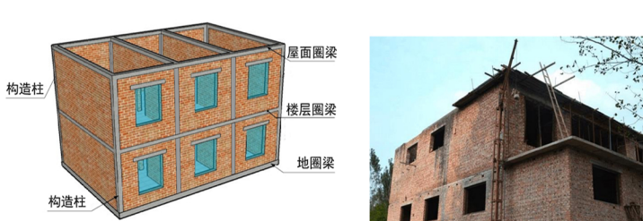
房屋设置圈梁、构造柱 (✓)
