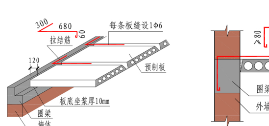
预制板端部与外墙拉结 (✓)
