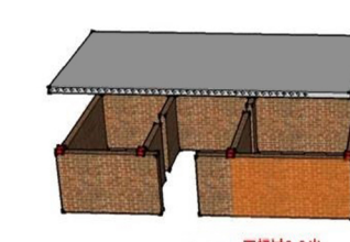
横墙间距不大于9米 (✓)
