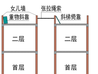
屋面女儿墙张拉绳索、重物倚靠 (✗)
