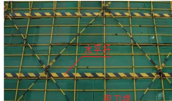
设置横杆、剪刀撑 (✓)
