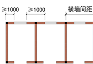
平面布置规整 (✓)
