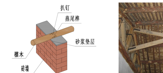
相邻檩木采用燕尾榫、扒钉连接 (✓)
