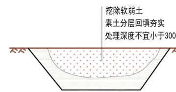
软弱土层进行地基处理 (✓)
